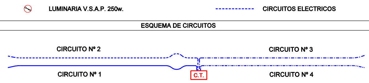
LEYENDA DE CIRCUITOS DE ALUMBRADO PUBLICO
