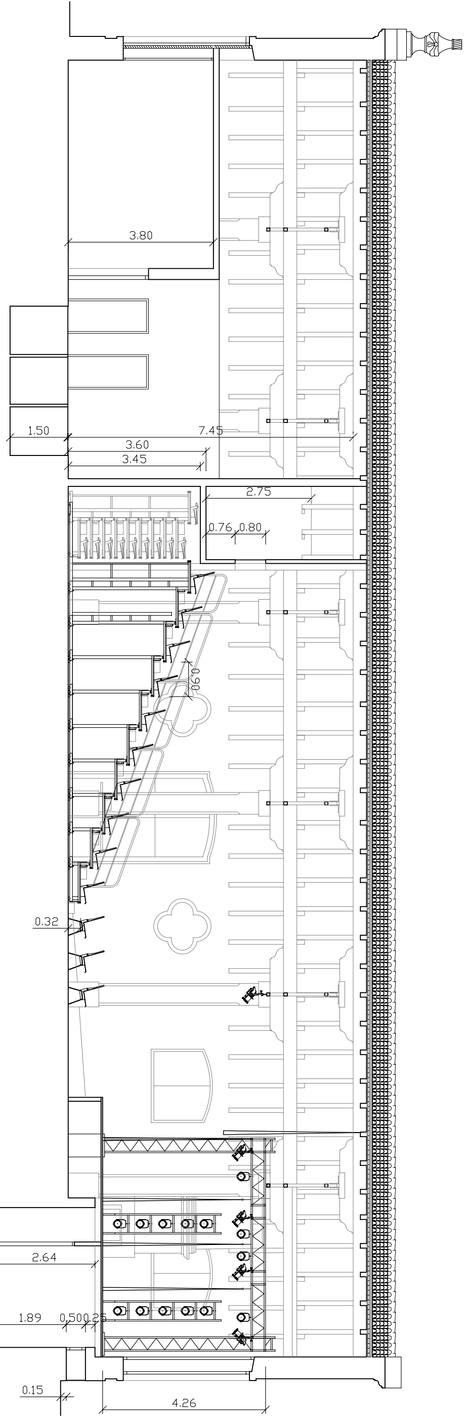
SECCION TRANSVERSAL
