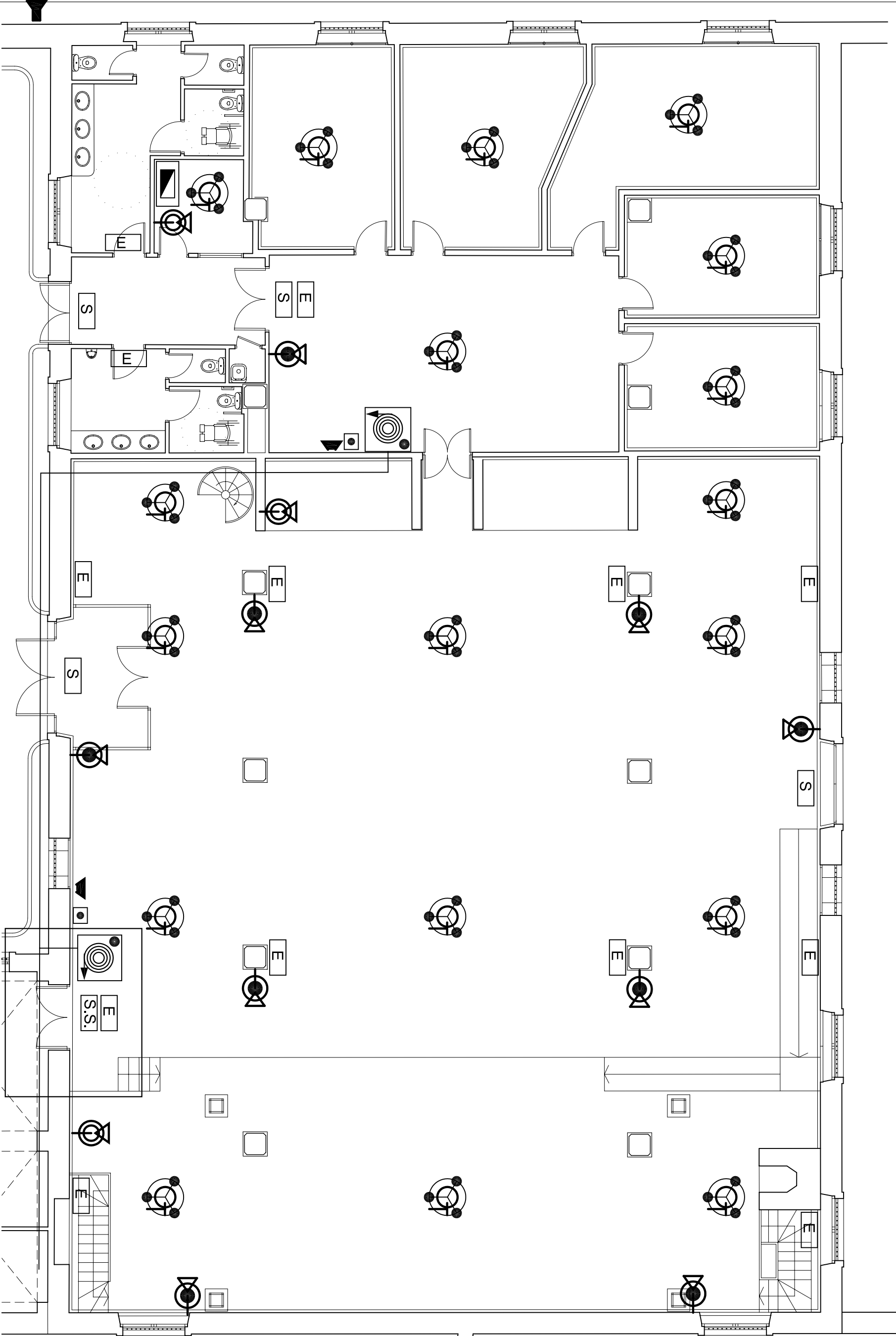
INSTALACION ELECTRICA
