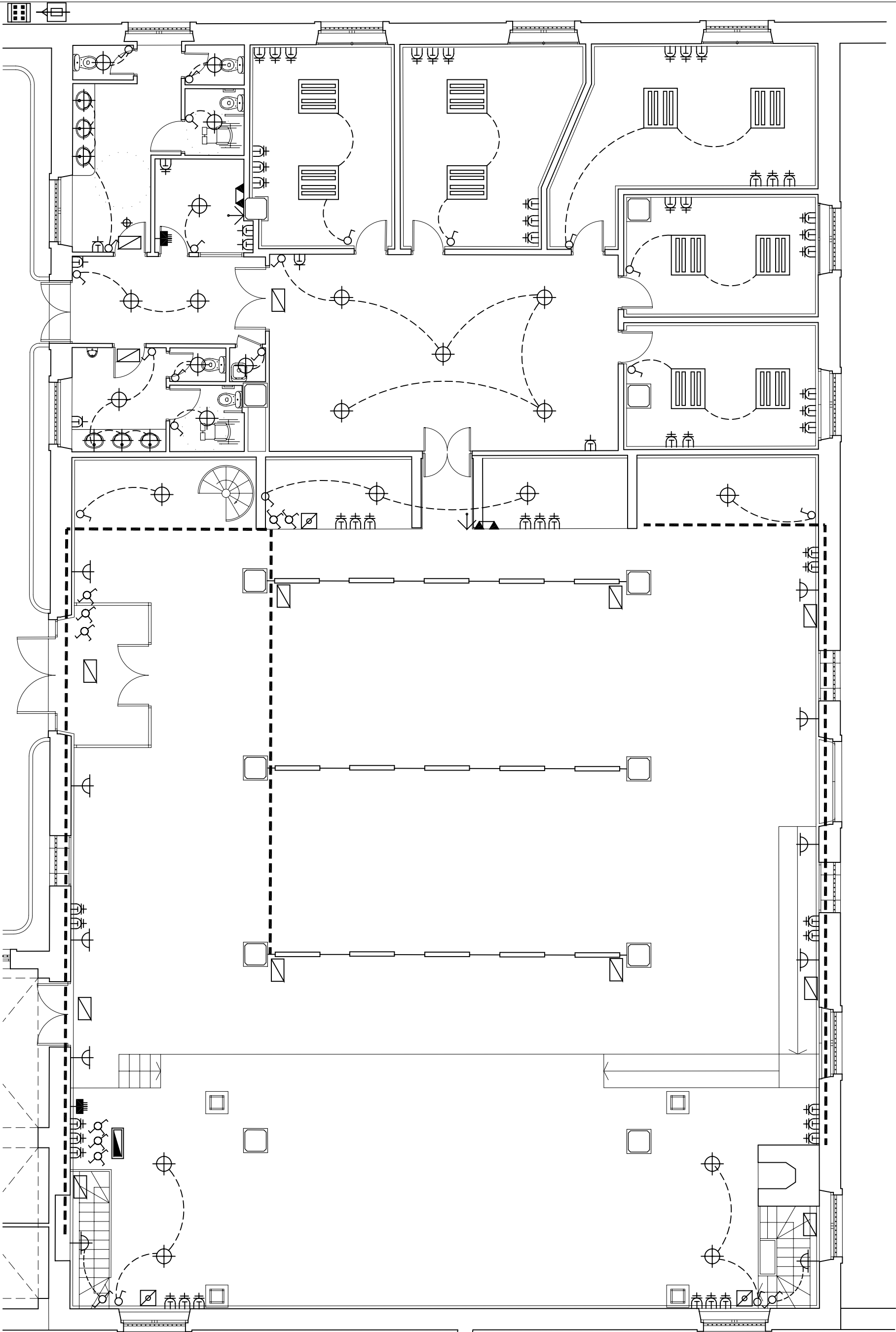
INSTALACION ELECTRICA
