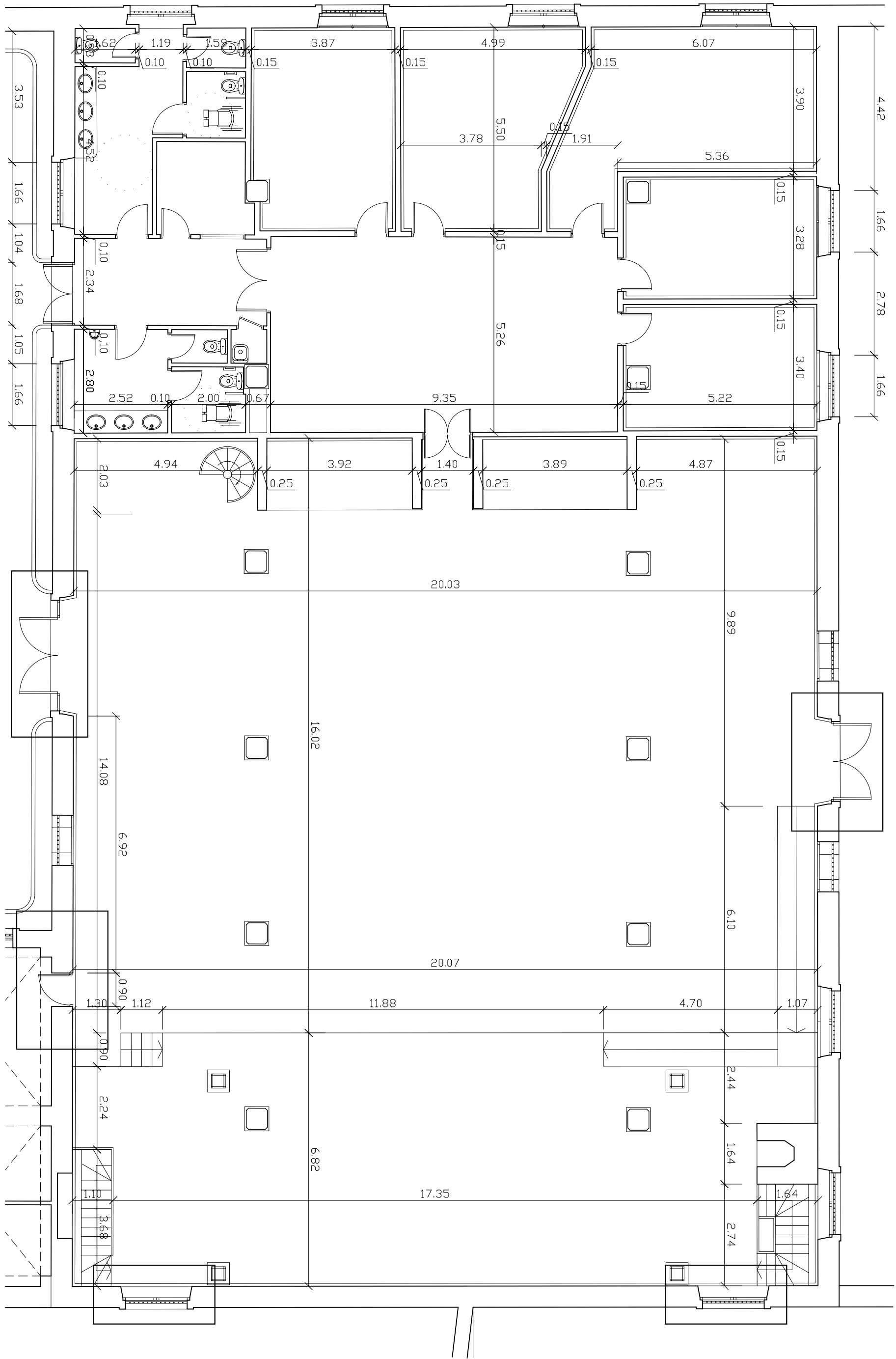
PLANTA DISTRIBUCION - ESTADO ACTUAL
