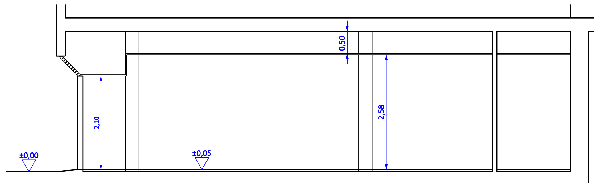
SECCIÓN REFORMADA
