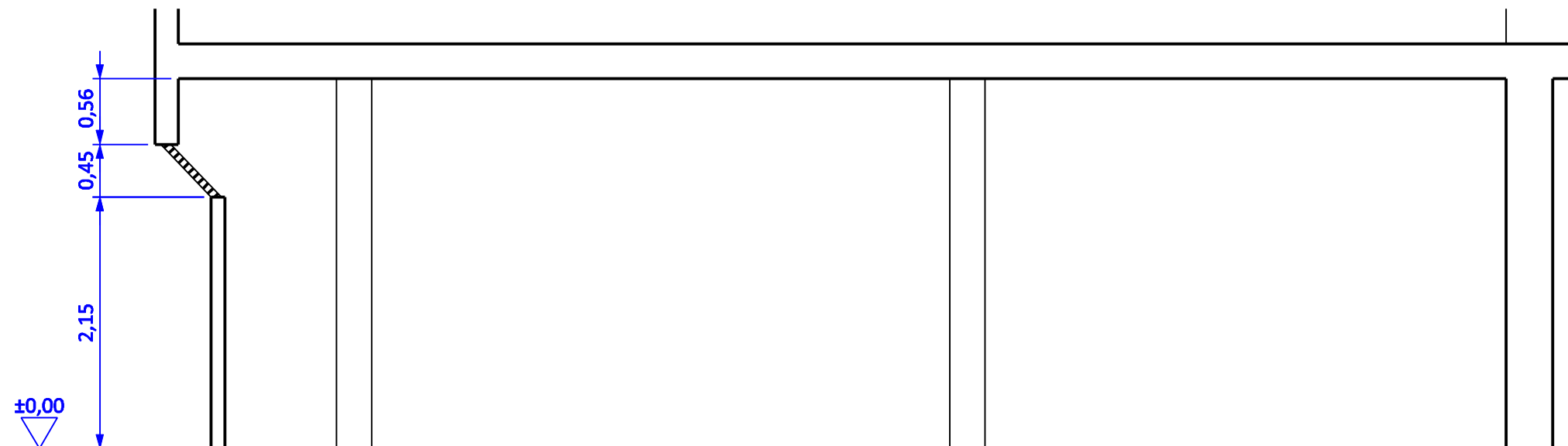
SECCIÓN ACTUAL
