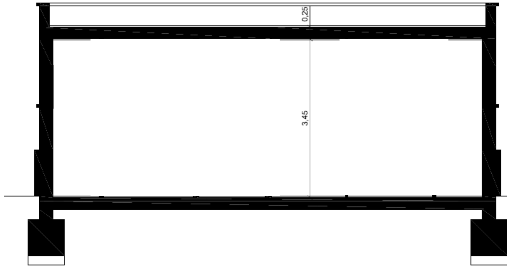
SECCION A-A
