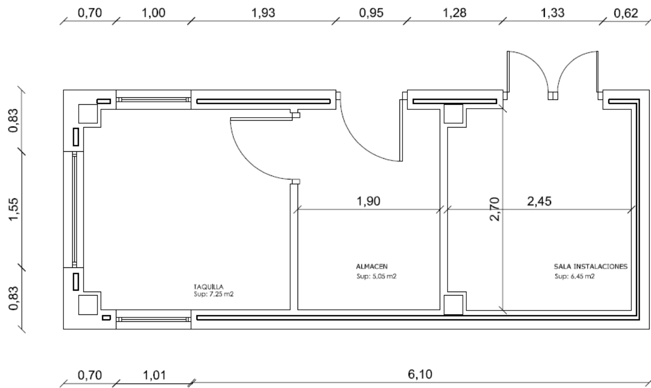
PLANTA DISTRIBUCIÓN
