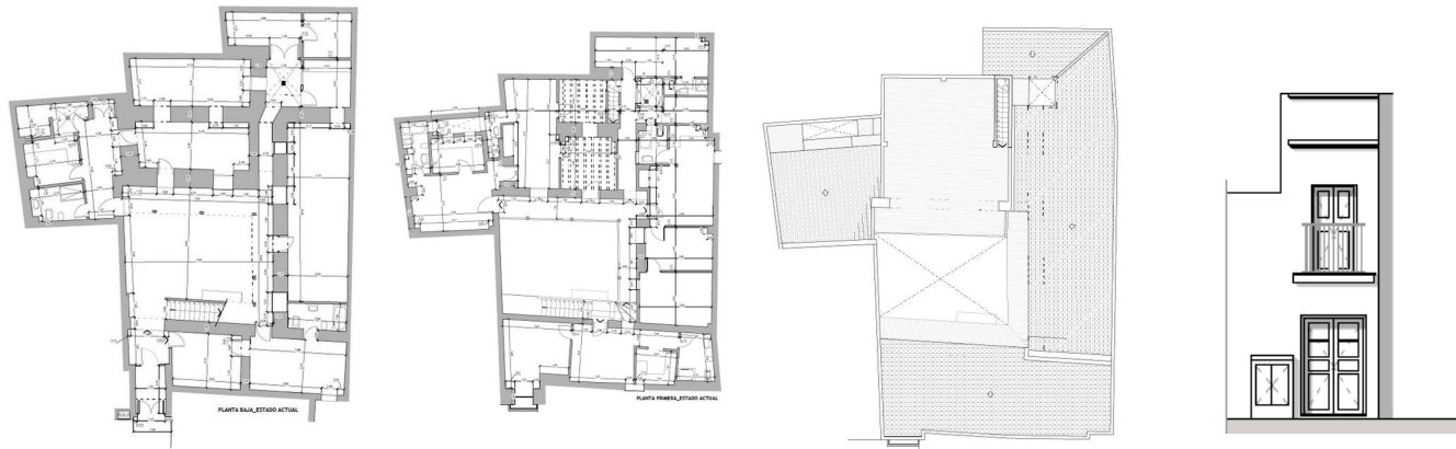
Planta Baja
